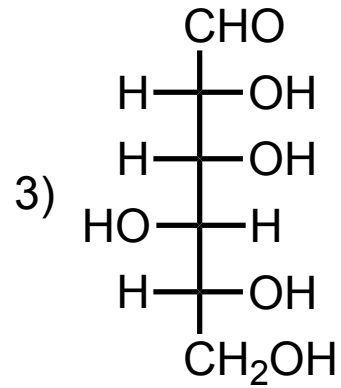
Gulose
