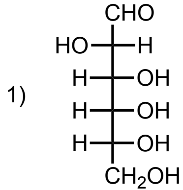
Altrose
