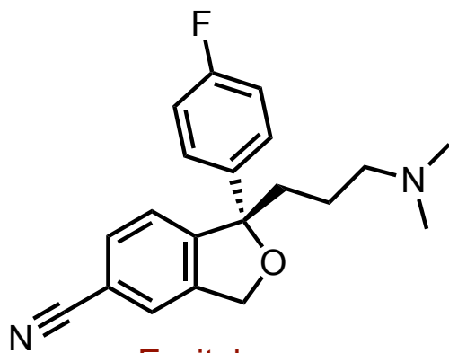
Escitalopram
