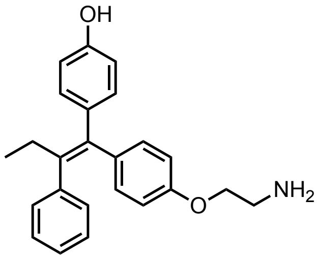
Norendoxifen
