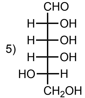
Talose
