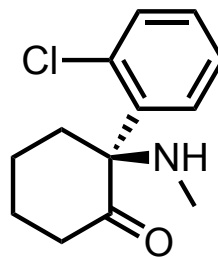
Esketamine
